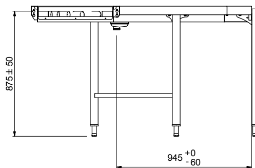
Zepředu
