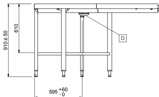
Boční
